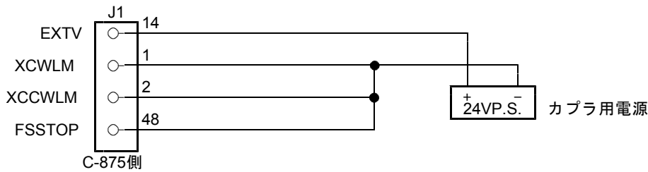
(1) LIMIT未使用時のX軸接続例
