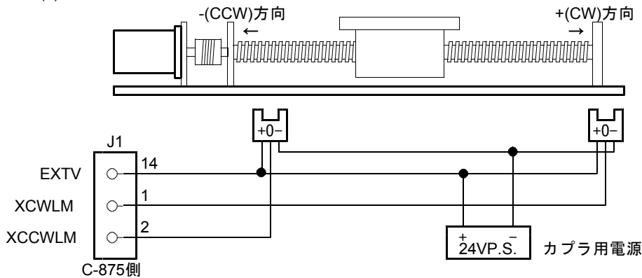
(2) LIMIT使用時のX軸接続例
