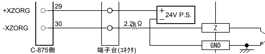
(注4)SERVO DRIVERのエンコーダZ相出力がオープンコレクタ出力の場合の接続例
